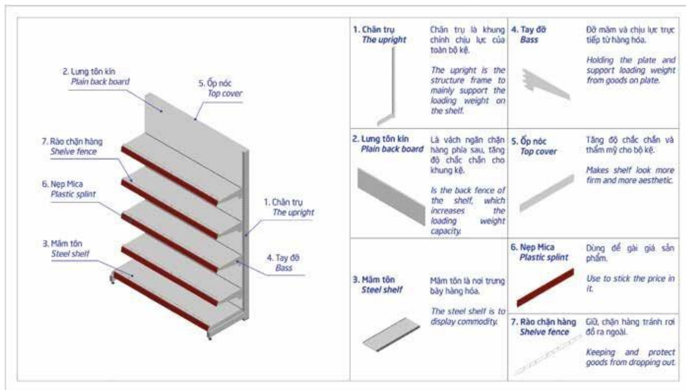
Cấu tạo kệ siêu thị Structure of supermarket shelves
