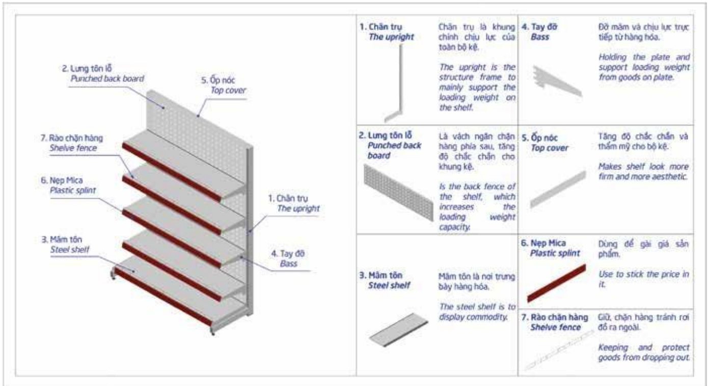
Cấu tạo kệ siêu thị Structure of supermarket shelves
